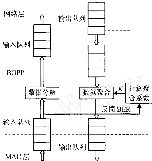
图 2 BGPP 的数据聚集机制
