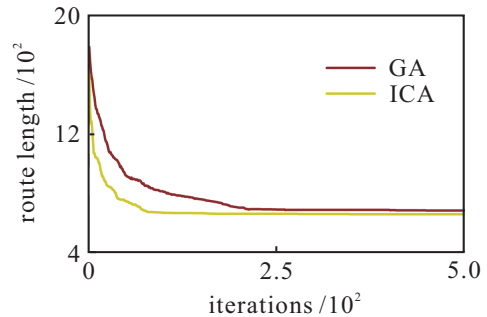
图8 ch150实例ICA与GA路径随迭代次数变化曲线
