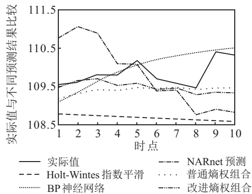
图4 汇率实际值与不同预测结果对比
