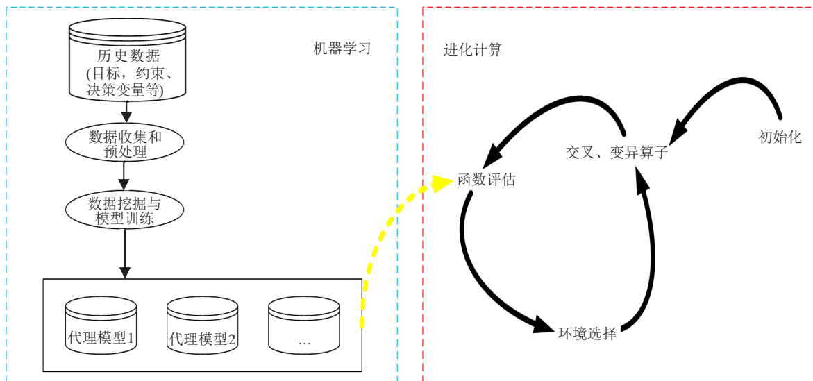
图4 数据驱动进化优化过程
