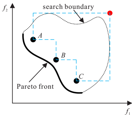
图10 HV指标几何意义
