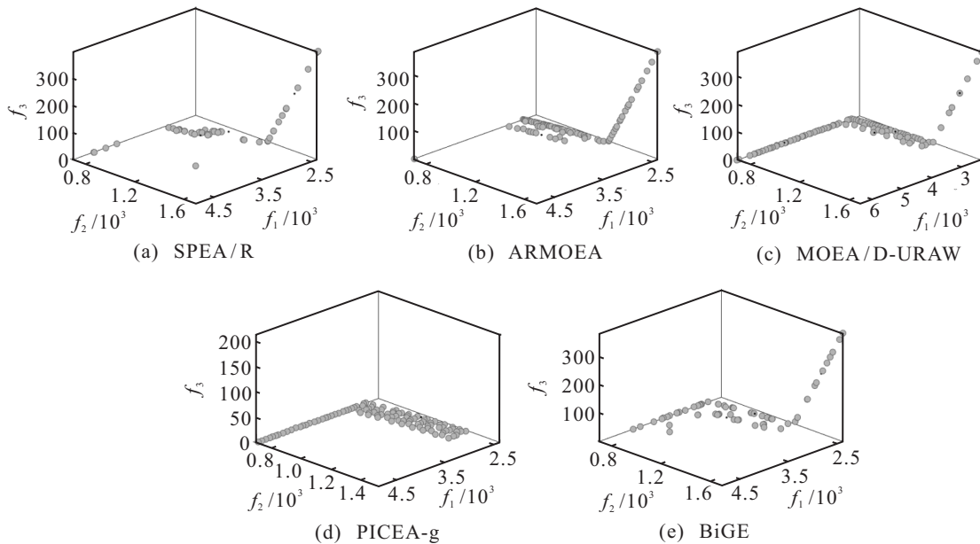
图 13 各算法在减速机设计问题上得到的非支配解集
