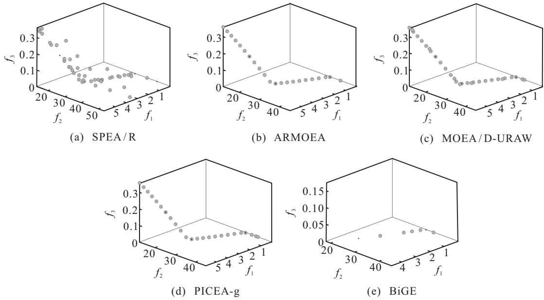
图 14 各算法在轮系设计问题上得到的非支配解集
