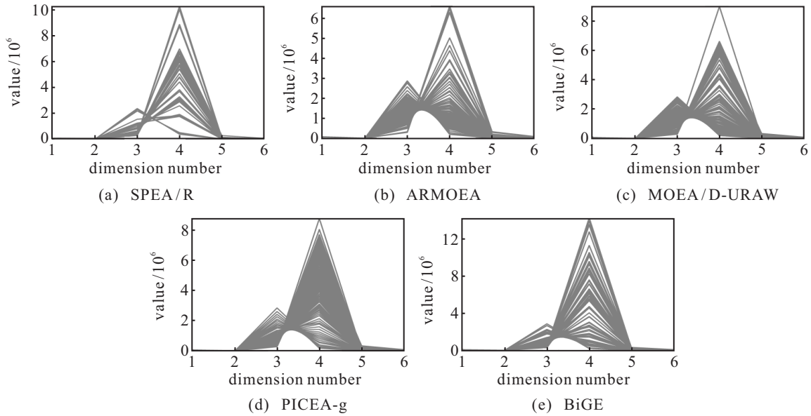
图 15 各算法在水资源规划问题上得到的非支配解集
