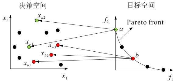
图3 多模态多目标优化问题目标空间与决策空间关系
