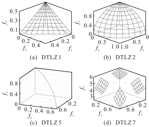
图8 DTLZ测试问题集中典型的Pareto前沿(3目标)
