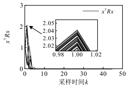
(b) 闭环系统
